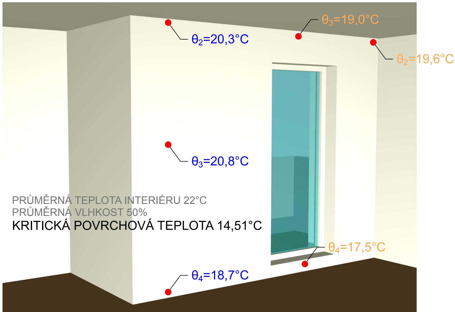
ZOBRAZENÍ NEJNIŽŠÍCH POVRCHOVÝCH TEPLOT V BYTOVÉM DOMĚ ULICE ČEŇKA RŮŽIČKY, BOHUNICE
